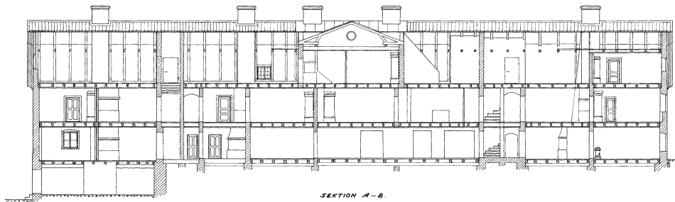
SEKTION A-B.
