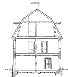
SEKTION C-D.
