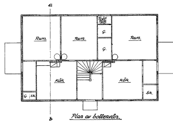
Plan av bottenvåning
