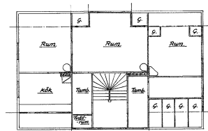
Plan av vindsvåning
