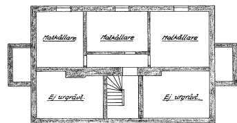
Källarplan
