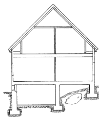
Sektion a-b
