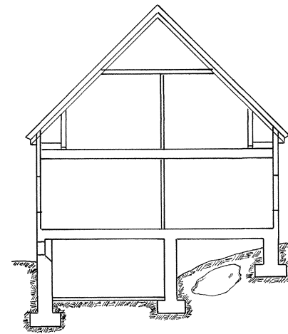
Sektion a-b.
